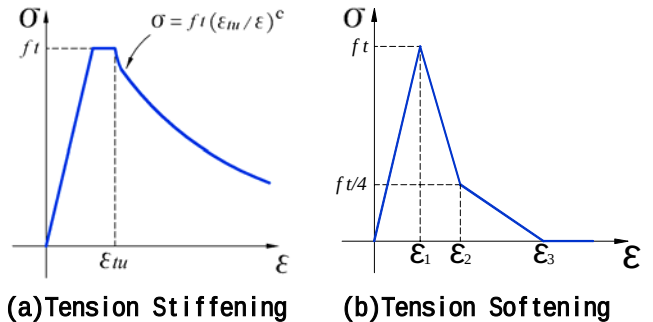
図-3 コンクリートの引張軟化特性
